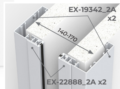
Perfiles puerta corredera en casetón
