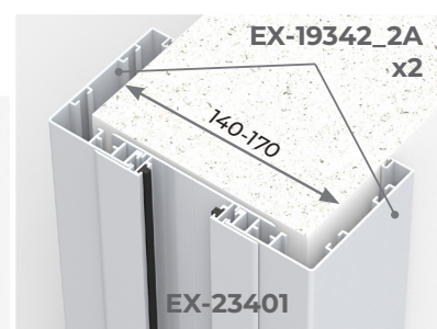
Perfiles puerta corredera batiente
