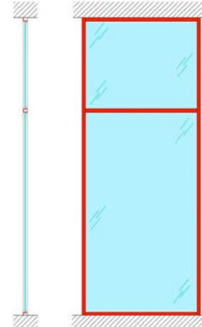
MAMPARA MONOPANEL SERIE MC45 - MÓDULO 08
