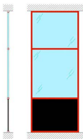
MAMPARA MONOPANEL SERIE MC45 - MÓDULO 09
