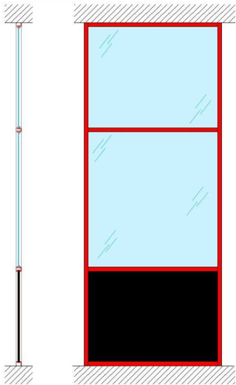
MAMPARA MONOPANEL SERIE MC45 MÓDULO 09
