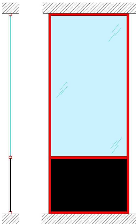
MAMPARA MONOPANEL SERIE MC45 MÓDULO 07
