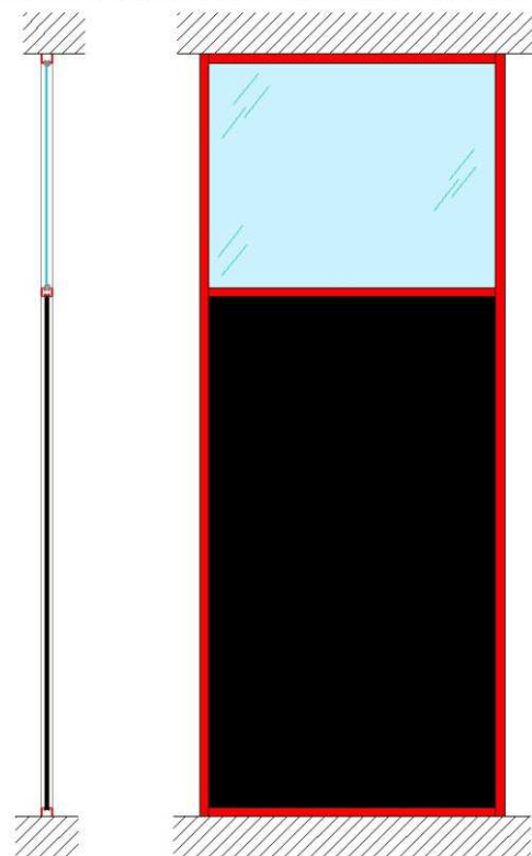
MAMPARA MONOPANEL SERIE MC45 MÓDULO 08
