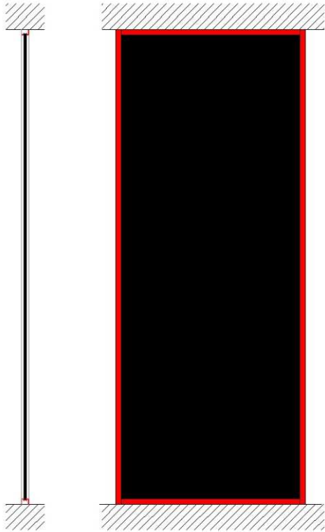
MAMPARA MONOPANEL SERIE MC45 MÓDULO 03
